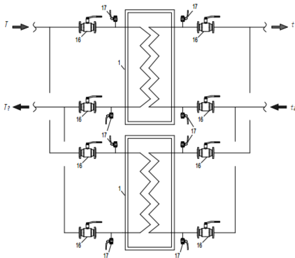
Схема резервирования водоподогревателя системы отопления
