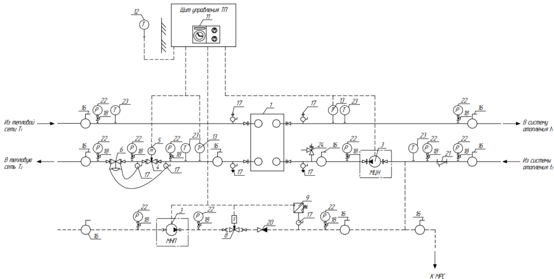
Технологическая схема №1 ИТП для одной системы отопления при независимом присоединении к тепловой сети
