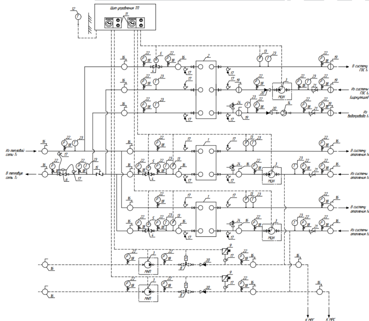
Технологическая схема №11а
