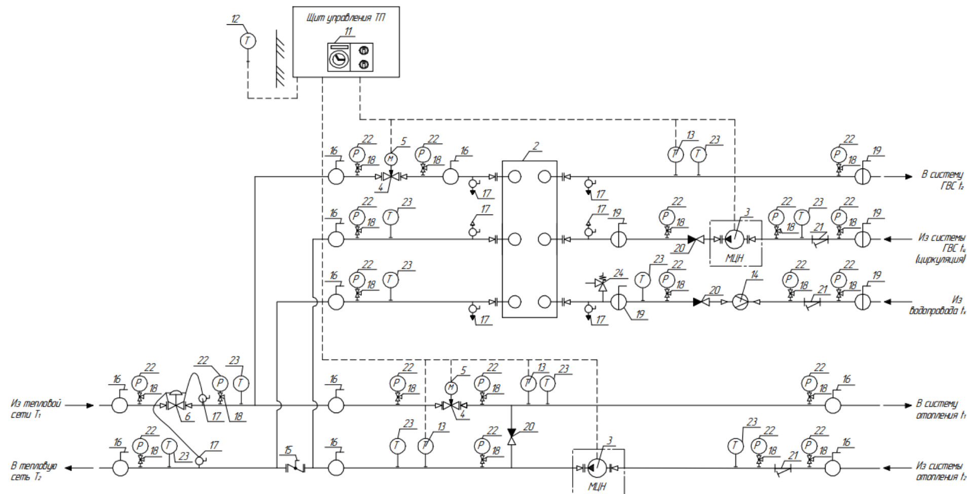
Технологическая схема №12а
