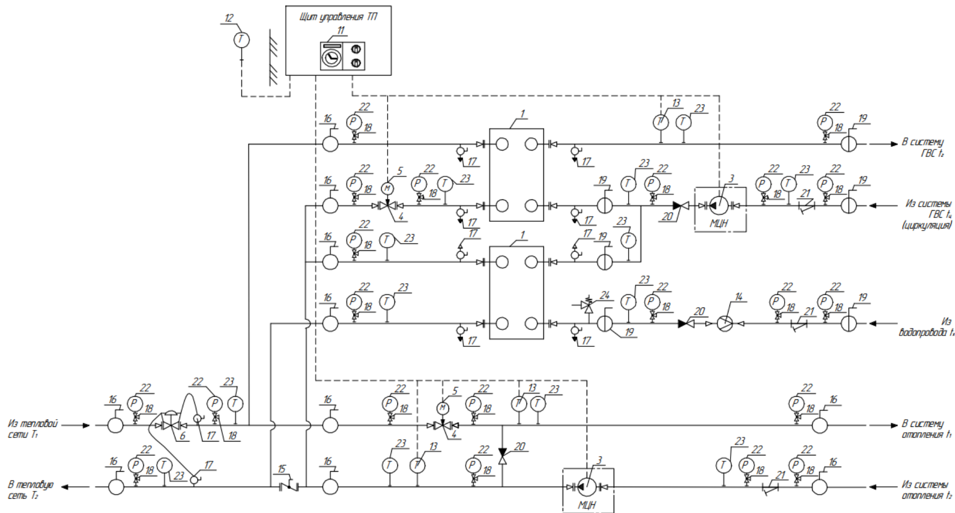
Технологическая схема №126
