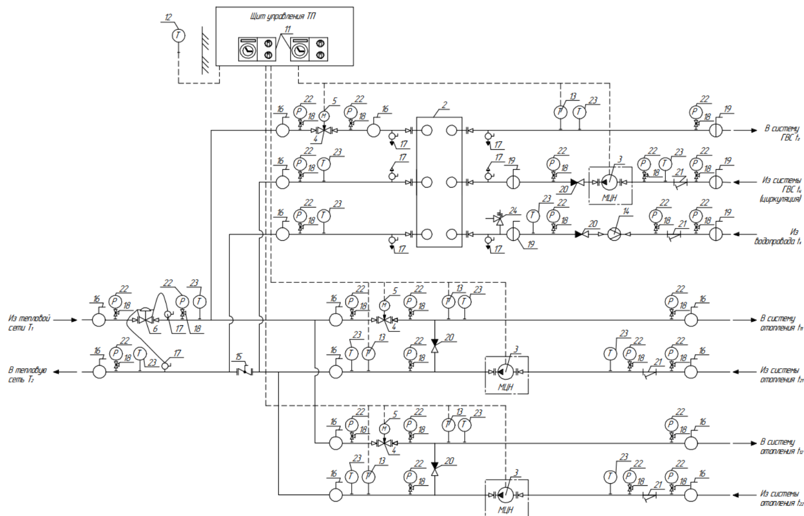
Технологическая схема №13а
