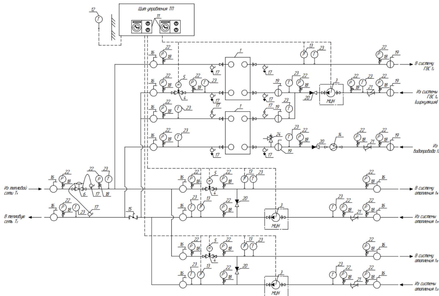
Технологическая схема №136
