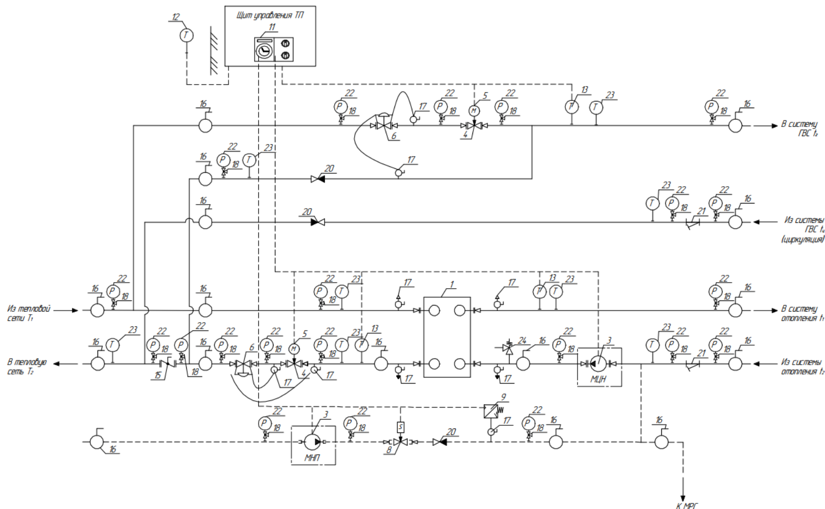
Технологическая схема №14
