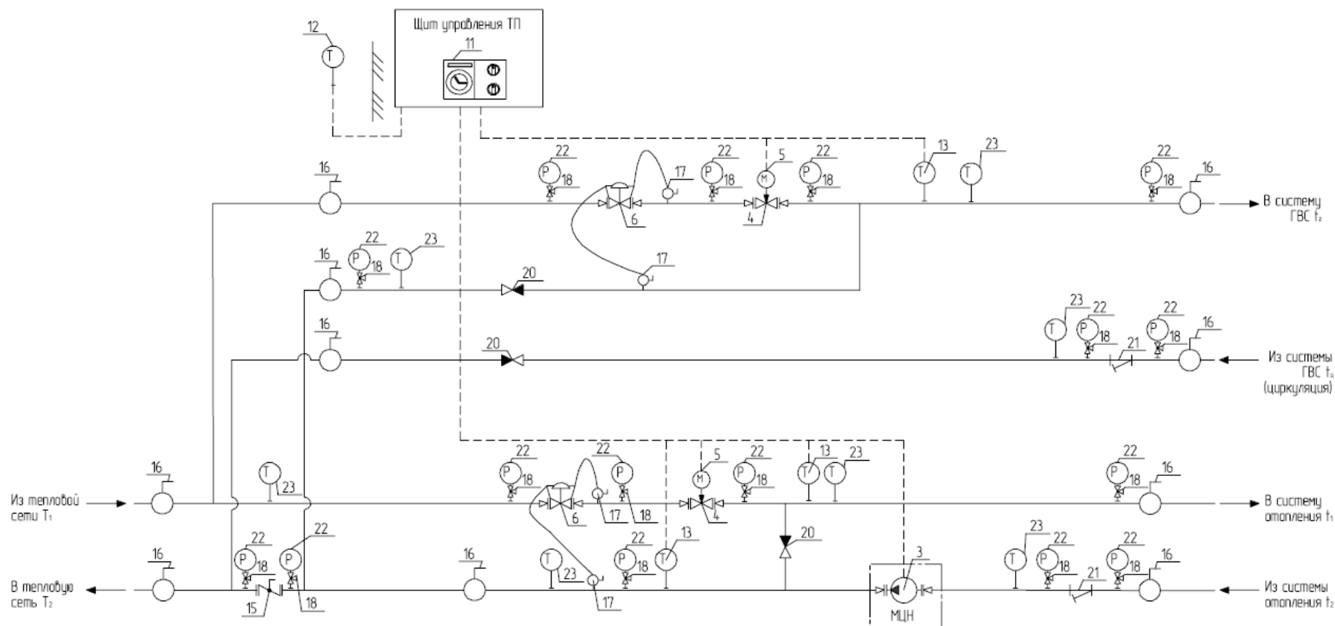
Технологическая схема №16
