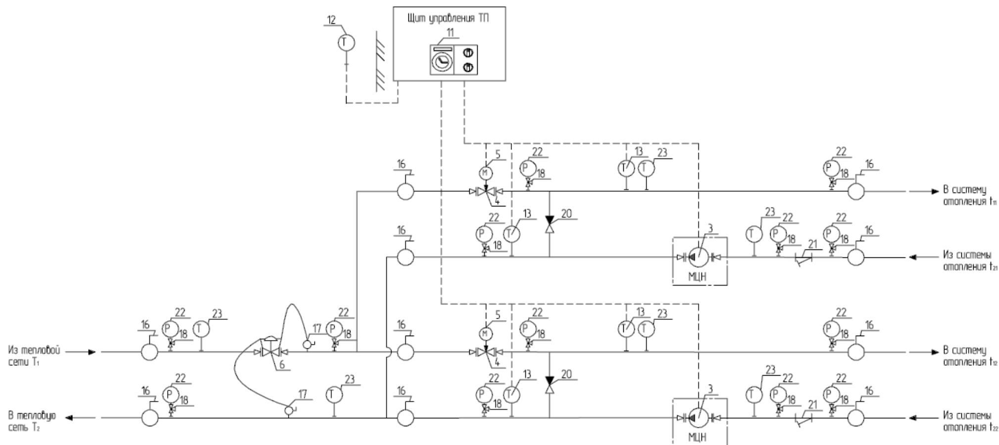
Технологическая схема №4 ИТП для двух систем отопления при зависимом присоединении к тепловой сети
