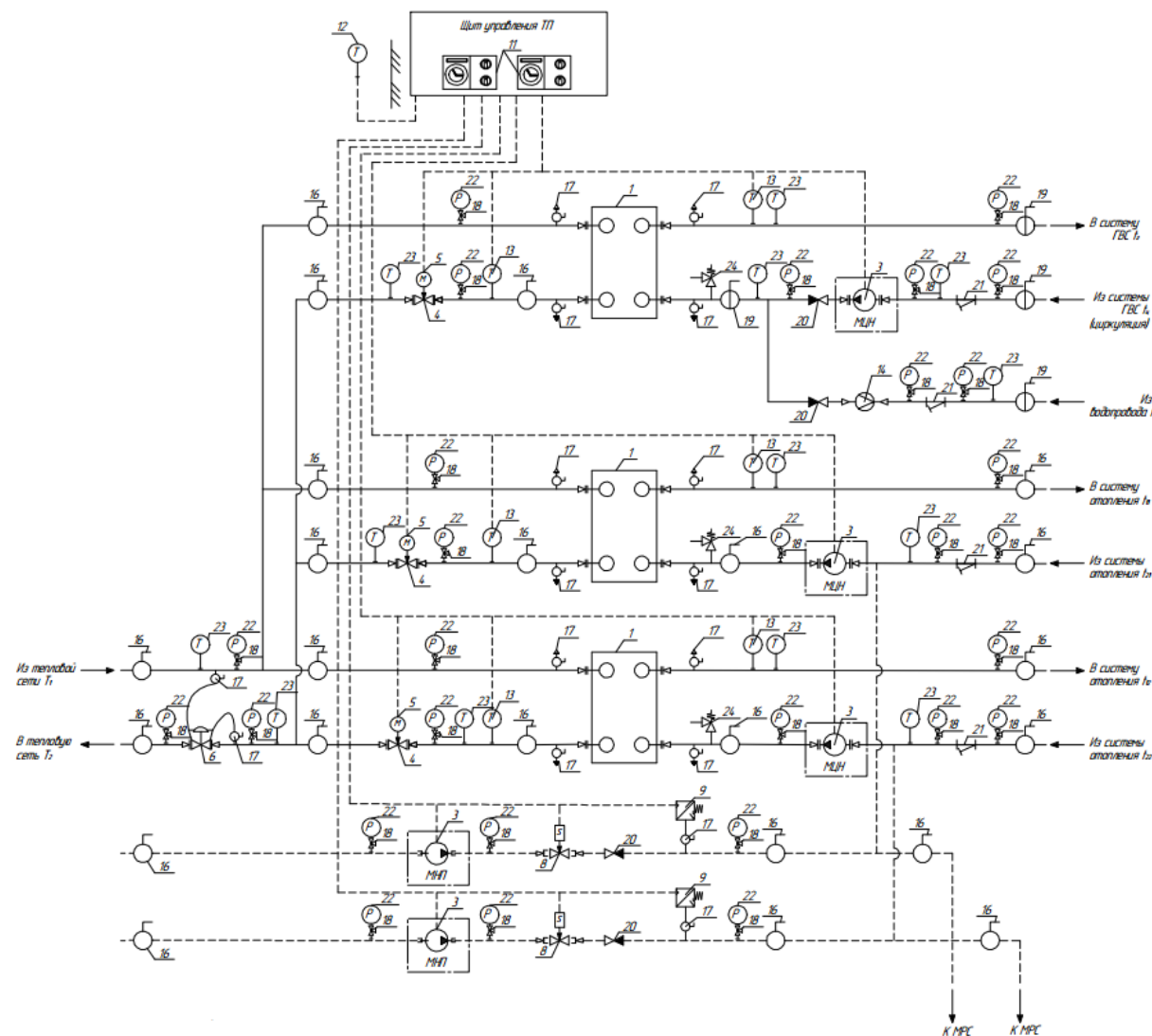
Технологическая схема №7
