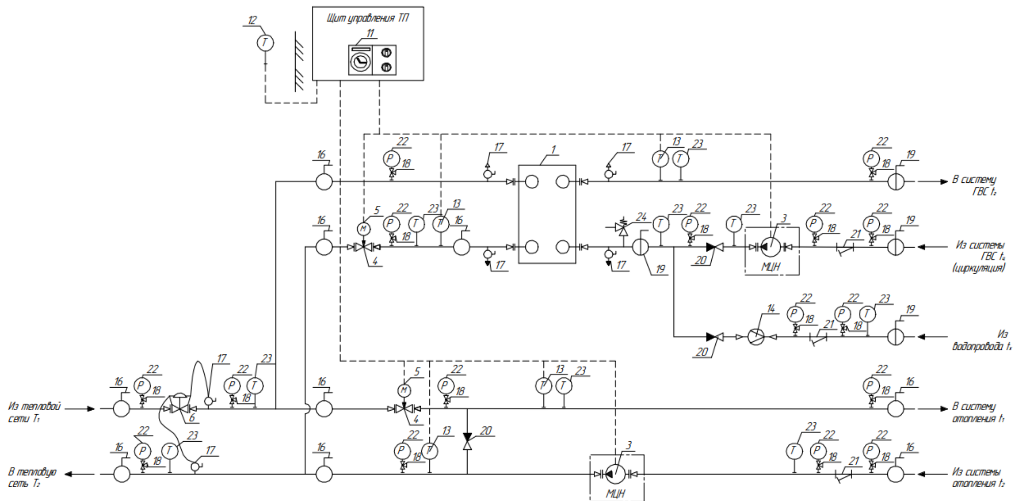
Технологическая схема №8
